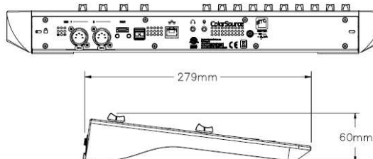
COLORSOURCE 20AV
