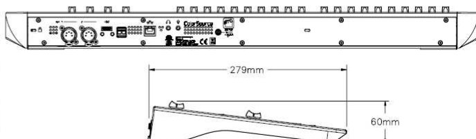
COLORSOURCE 40AV
